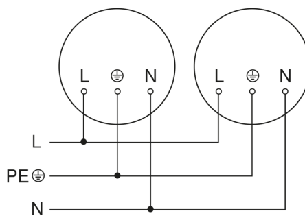
Schéma du circuit
