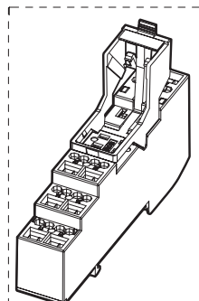
Optie (met bijgevoegde uitwerper en label)
