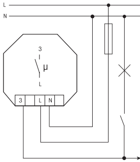
überwachter Stromkreis
