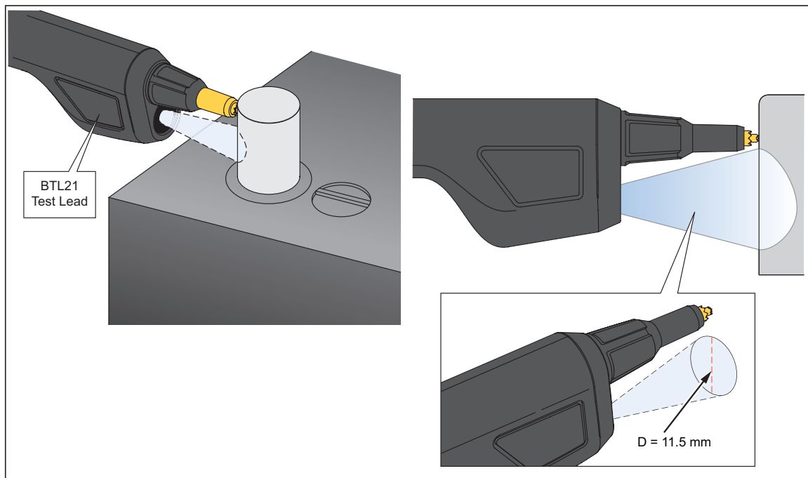
Afbeelding 4-5. De temperatuur van een batterijpool meten
