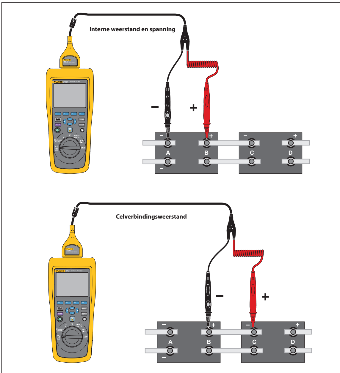
Afbeelding 3-1. De interne weerstand en de spanning van een batterij meten
