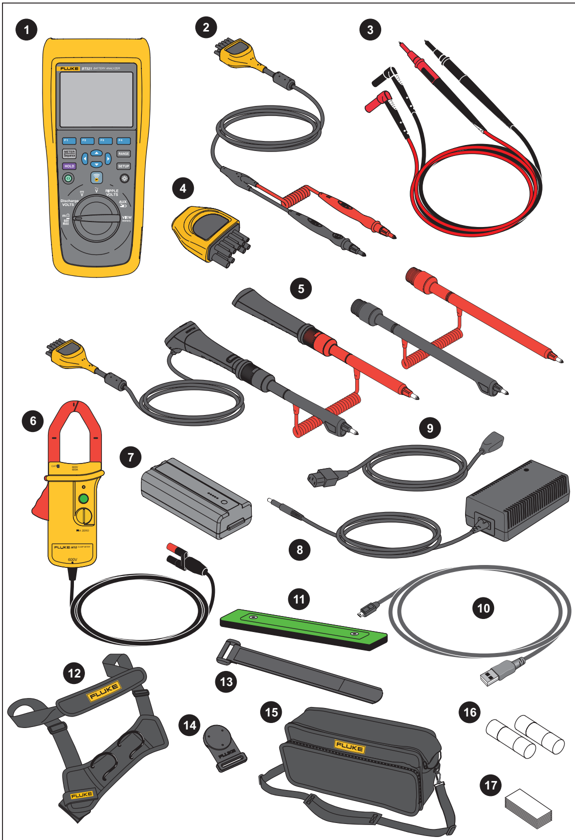
Abbeelding 1-1. Standaarduitrusting
