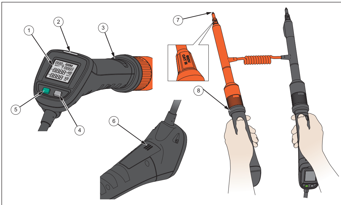
Afbeelding 4-1. BTL21 Interactive Test Probe
