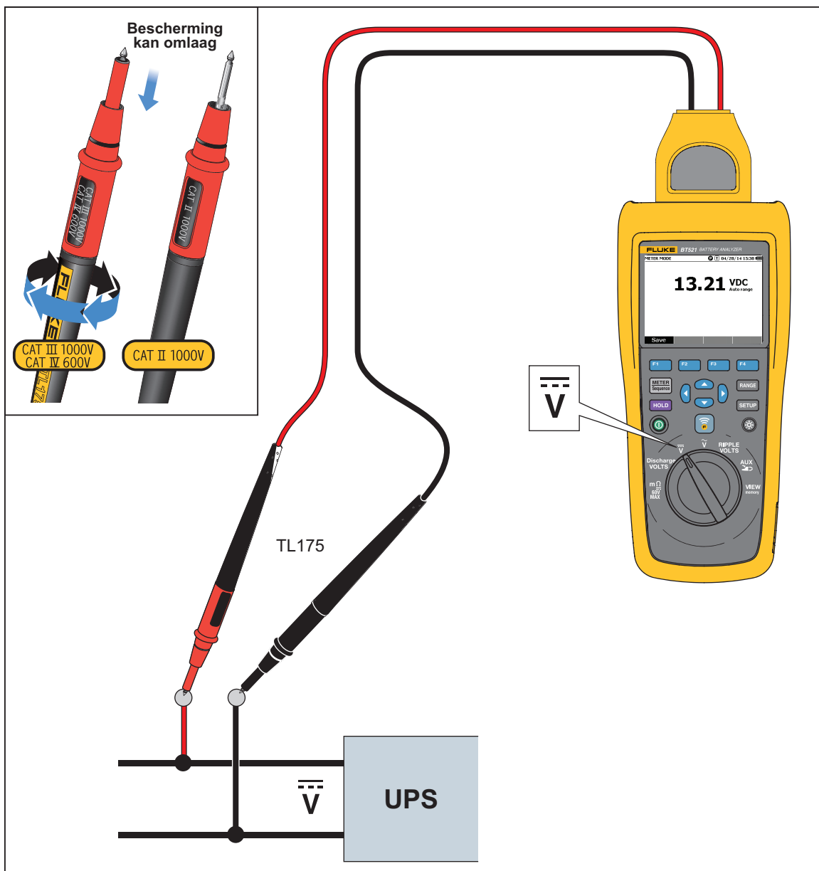
Afbeelding 3-6. DC-spanning meten met TL175
