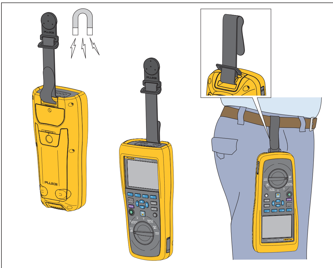
Afbeelding 2-2. De draagriem
