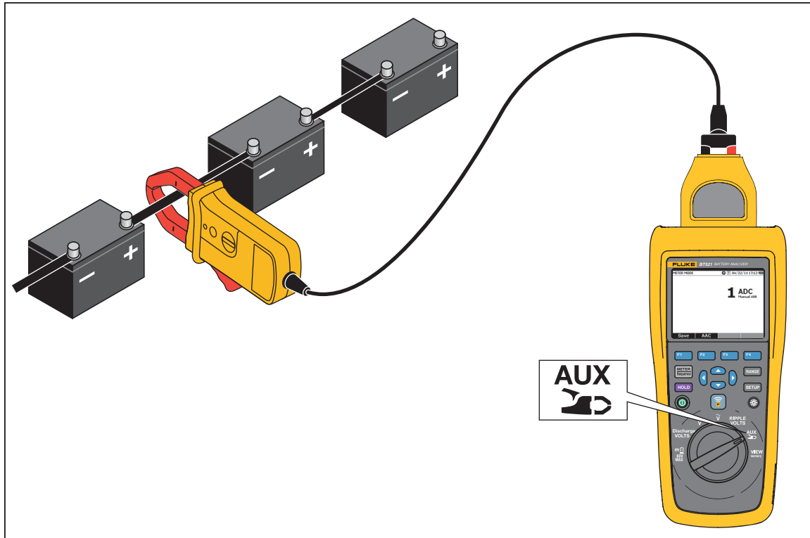
Afbeelding 3-5. AUX-functie
