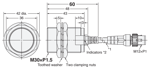
E2E-X10B4-M1TJ-IL□
