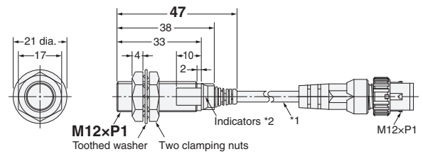
E2E-X3B4-M1TJ-IL□
