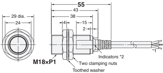
E2E-X7B4-IL□
