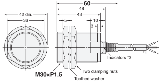
E2E-X10B4-IL□
