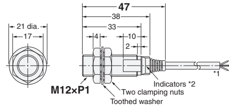
E2E-X3B4-IL□
