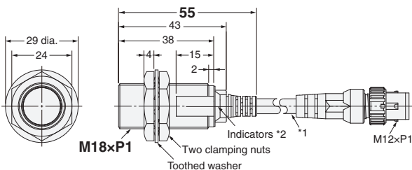
E2E-X7B4-M1TJ-IL□
