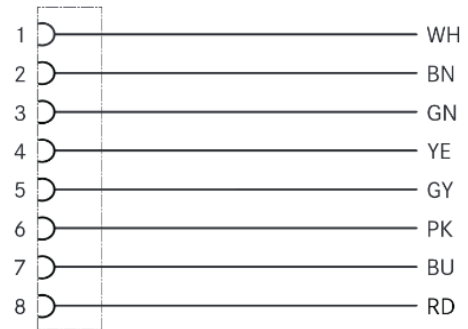
Cable
