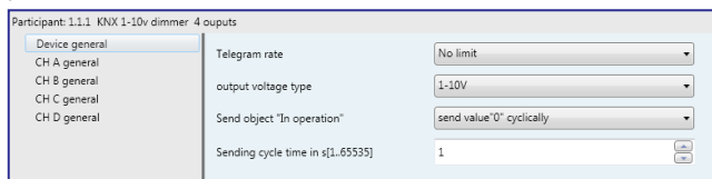
Fig. 6.1 Parameter window "Device general"
