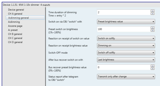
Fig. 6.4 Parameter window "CH X dimming general"
