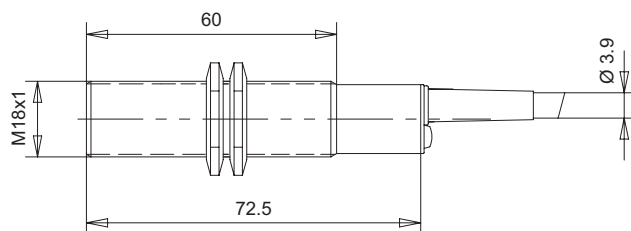
E2F-DX8M□-L 2M
