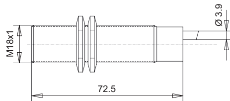
E2F-DX8M□-L 2M
