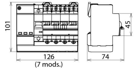
Dimension drawing SPD+POP 4 255 C40
