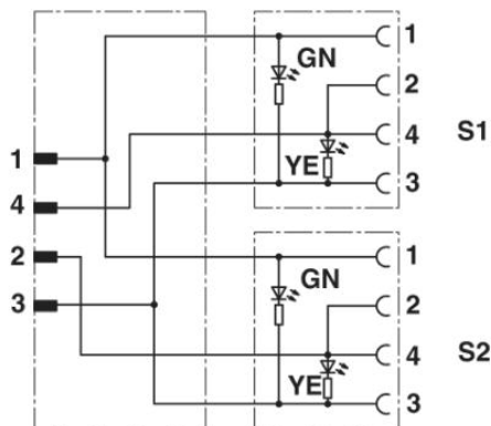
Schaltplan
