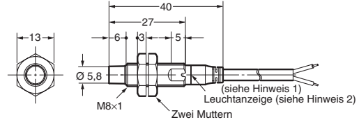
E2A-S08KN04-WP-□□
