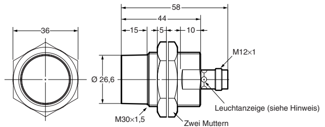
E2A-M30KN20-M1-□□/E2A-S30KN20-M1-□
