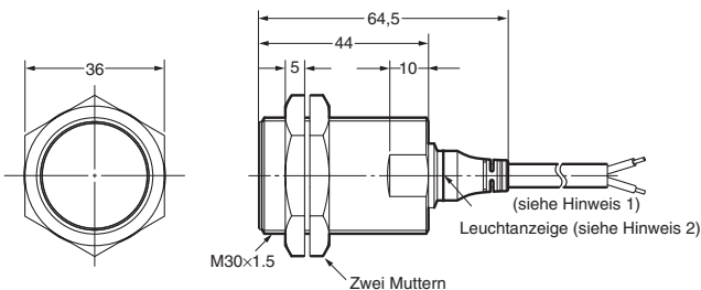
E2A-M30KS15-WP-□□/E2A-S30KS15-WP-□
