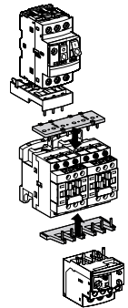
LAD9VP3 = LAD9V5 + LAD9V6
