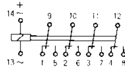
DIN-Schaltbild
