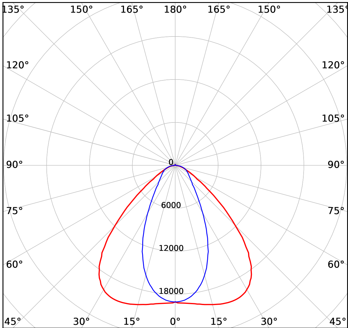
cd 32000 lm — C0-C180 — C90-C270
