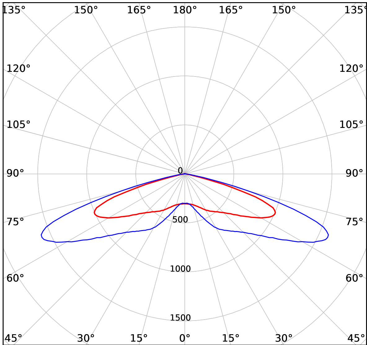
cd 4300 lm — C0-C180 — C90-C270
