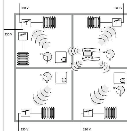
Bild 3: Zeitsteuerung mit Master- und Slavereglern
