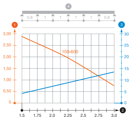
Slodzes diagramma, kabeļu rene, tips SKSMU 85
