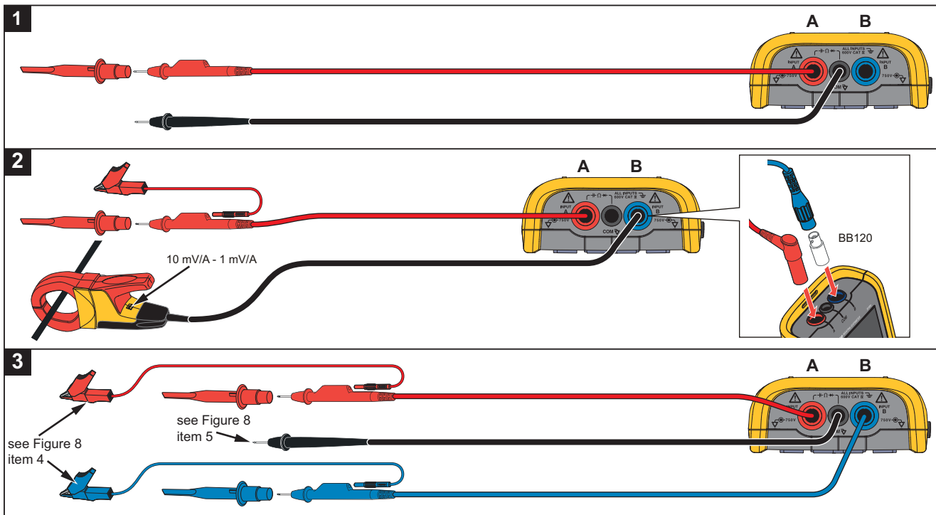
Afbeelding 7. Meetopstellingen
