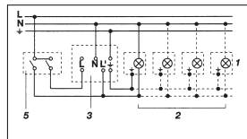
3. Conexão mediante comutador em série para modo manual e automático
