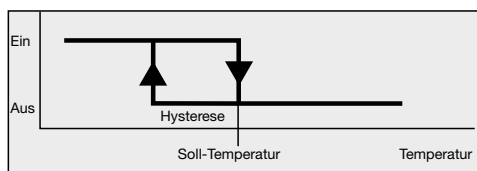
Bild 2: 2-Punkt-Regelung
