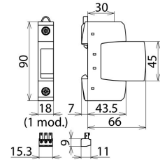
Dimension drawing DG SU 1P 347 R
