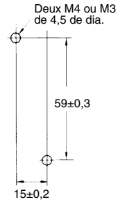
Trous de montage
