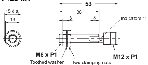
E2E-X□L12-M1
